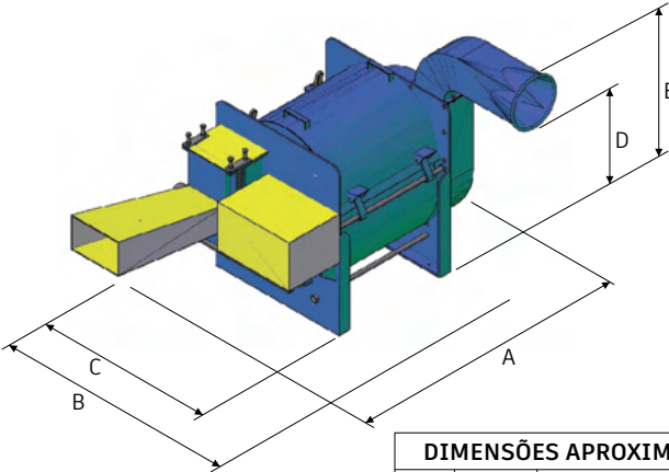
Ilustração 08 Desenho sem escala Perspectiva da Máquina com medidas aproximadas Empresa: São Ferreiro
