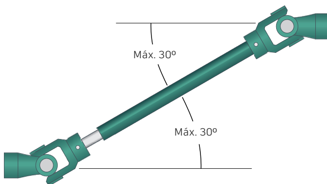
Ilustração 11 Ângulo máximo para alinhamento do eixo cardan
